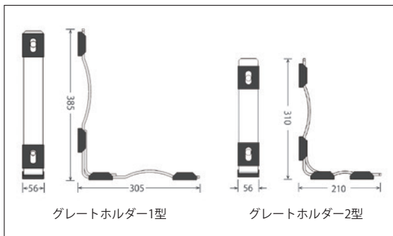
グレートホルダー1型（左）／2型（右）
