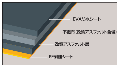
製品構造図
