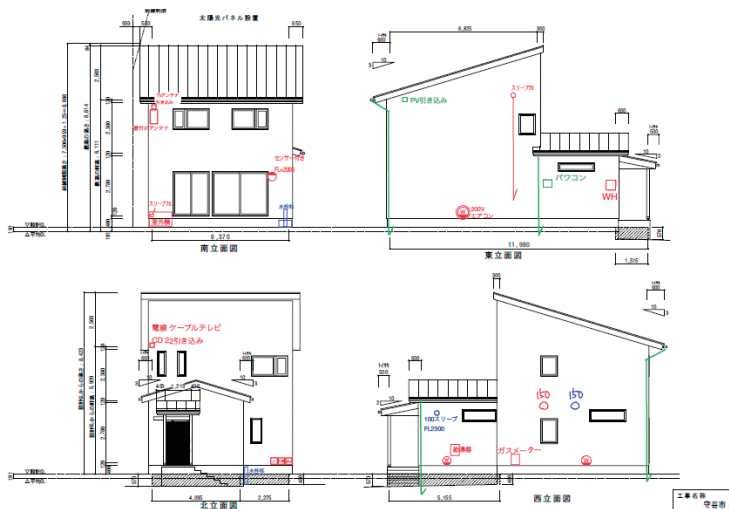
立面図
