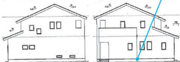
【西立面図】
