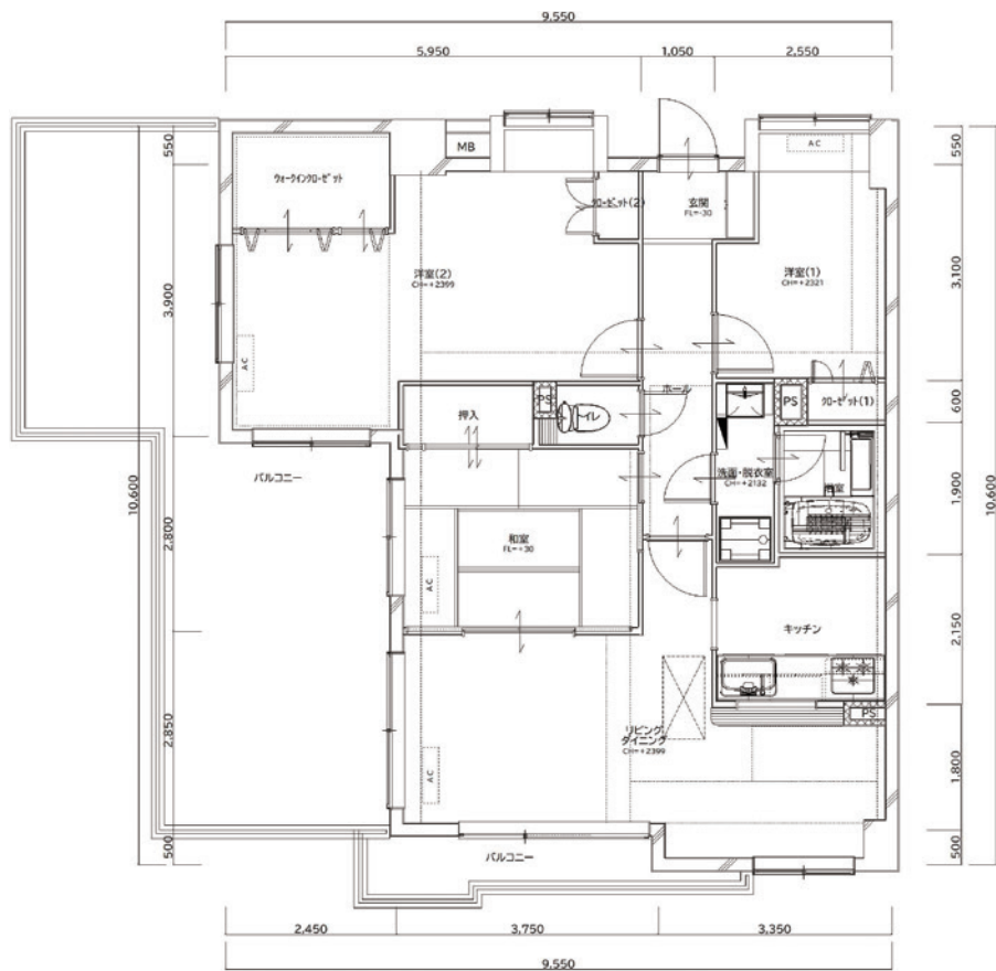
既存平面図
