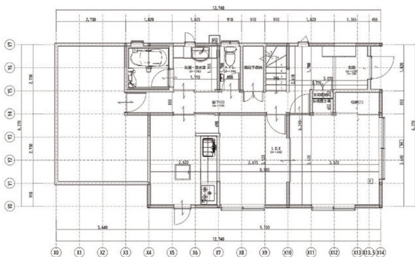
1階平面図
