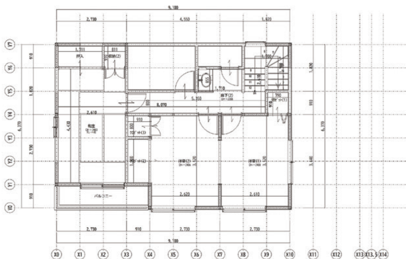
2階平面図
