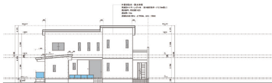
東側立面図
