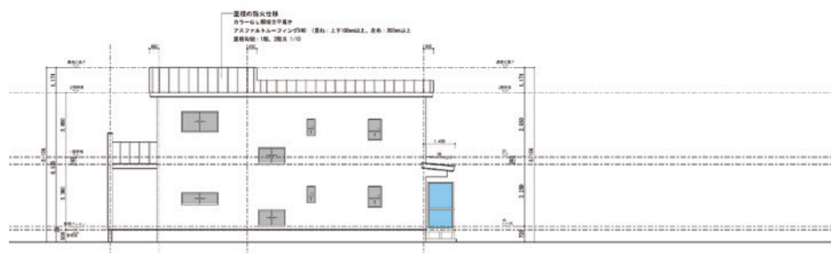
西側立面図
