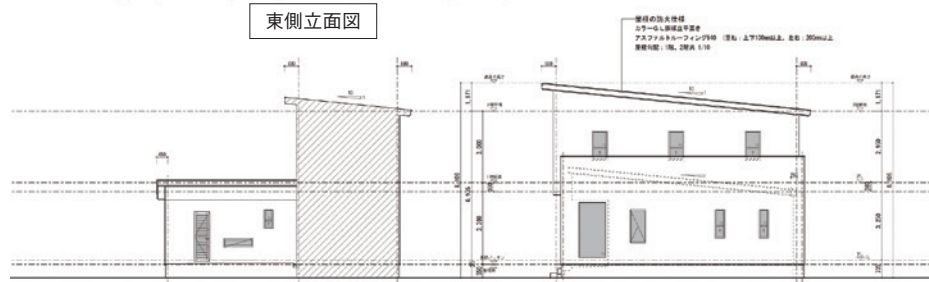
テラス北側立面図
