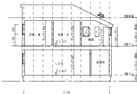
東西断面図 S:1/100
