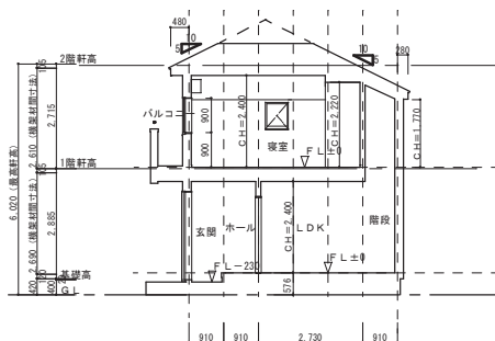
南北2 S:1/100
