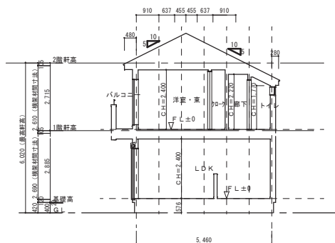
南北断面図 S:1/100
