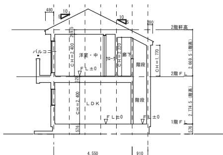
南北3 S:1/100
