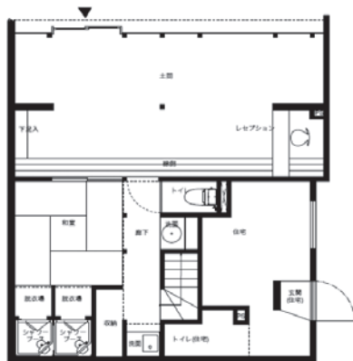
改修1階平面図 G=1/50
