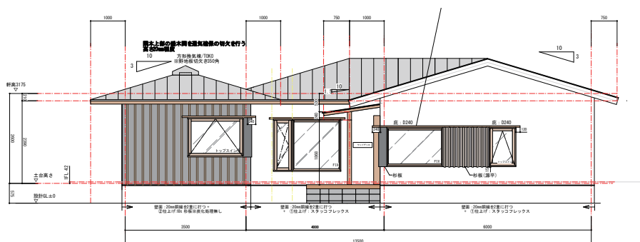
東立面図
