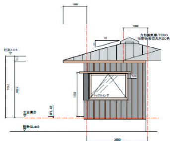
中庭 北立面図
