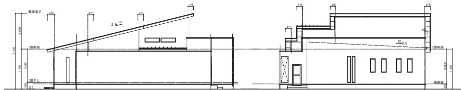
南側立面图 S : 1/100
