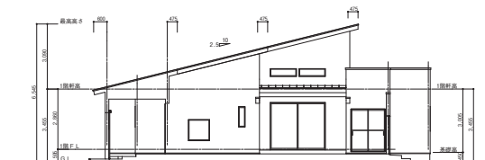
南側立面图 (堀内より) S : 1/100
