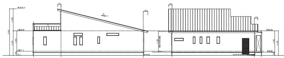
北側立面图 S : 1/100
