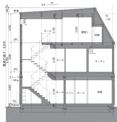
断面図-2 (X-X) S : 1/50
