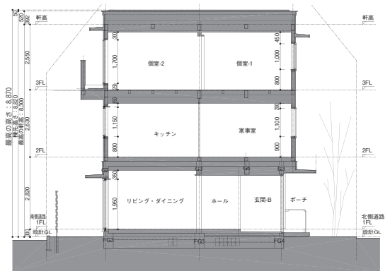
断面図-3 (Y-Y) S : 1/50
