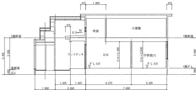
南北方向 断面图 S:1/100
