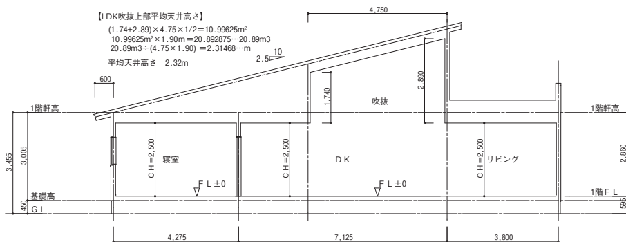
東西方向 断面図 S:1/100
