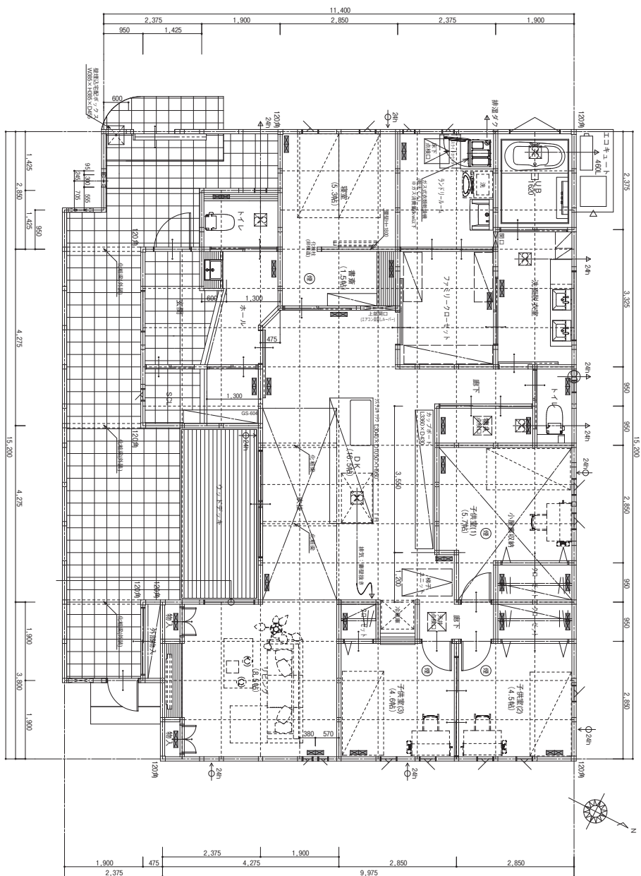
平面図
