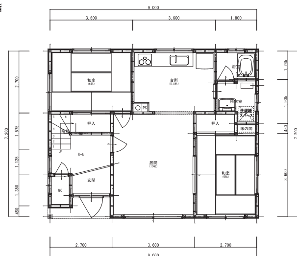
1階
