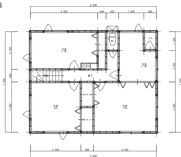
2階
