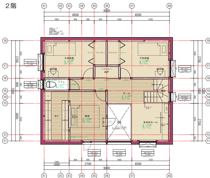
2階
