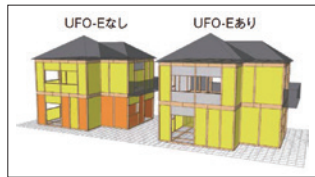
地震動を与えた場合の挙動をシミュレーション。オレンジ色の部分は損傷の恐れがあることを示している。
