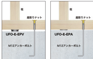
設置イメージ (2×4・剛床・根太レス床組み座彫りナット使用時)
