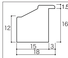
2250×16.0mmタイプ
