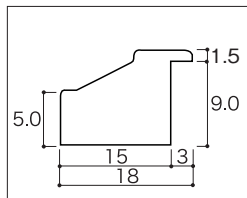
2250×9.0mmタイプ
