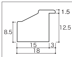
2250×12.5mmタイプ(1)
