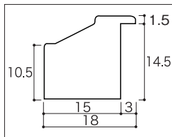
2250×14.5mmタイプ
