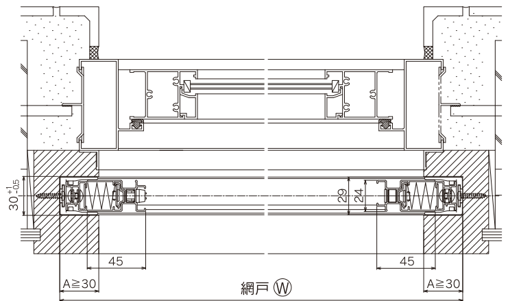
● 横断面図 ●
