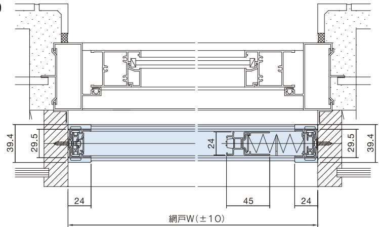
● 横断面納まり図 ●
