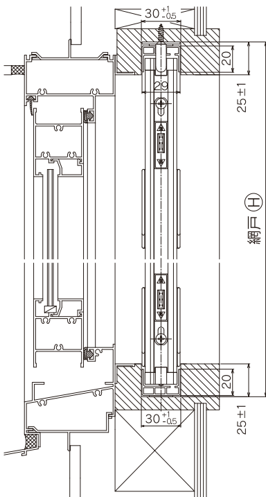
● 縦断面図 ●
