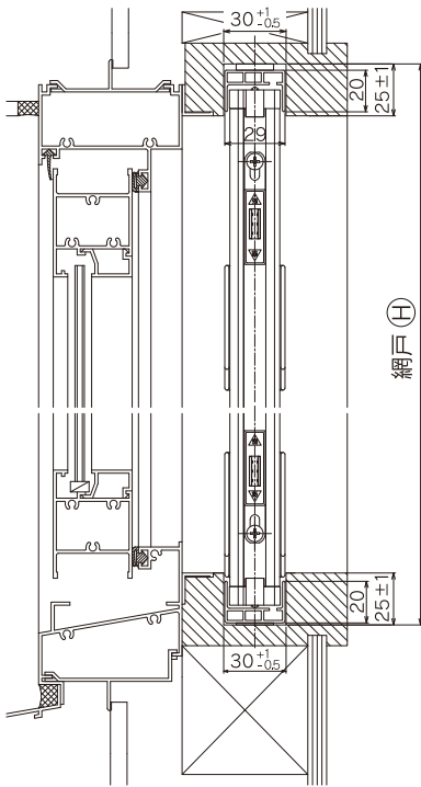
● 縦断面図 ●
