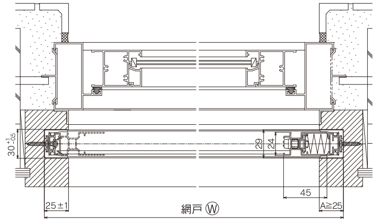
● 横断面図 ●
