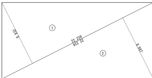
敷地面積求積図
