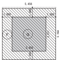
カーポート求積図
