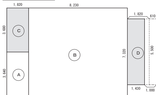
1階床面積求積図
