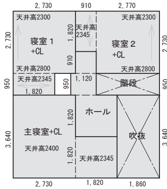
2階各室求積図
