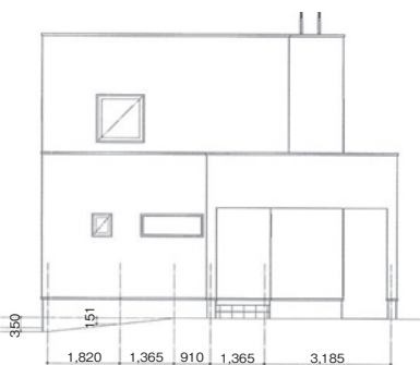
西側 立面図
