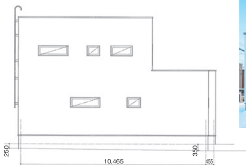
北側 立面図
