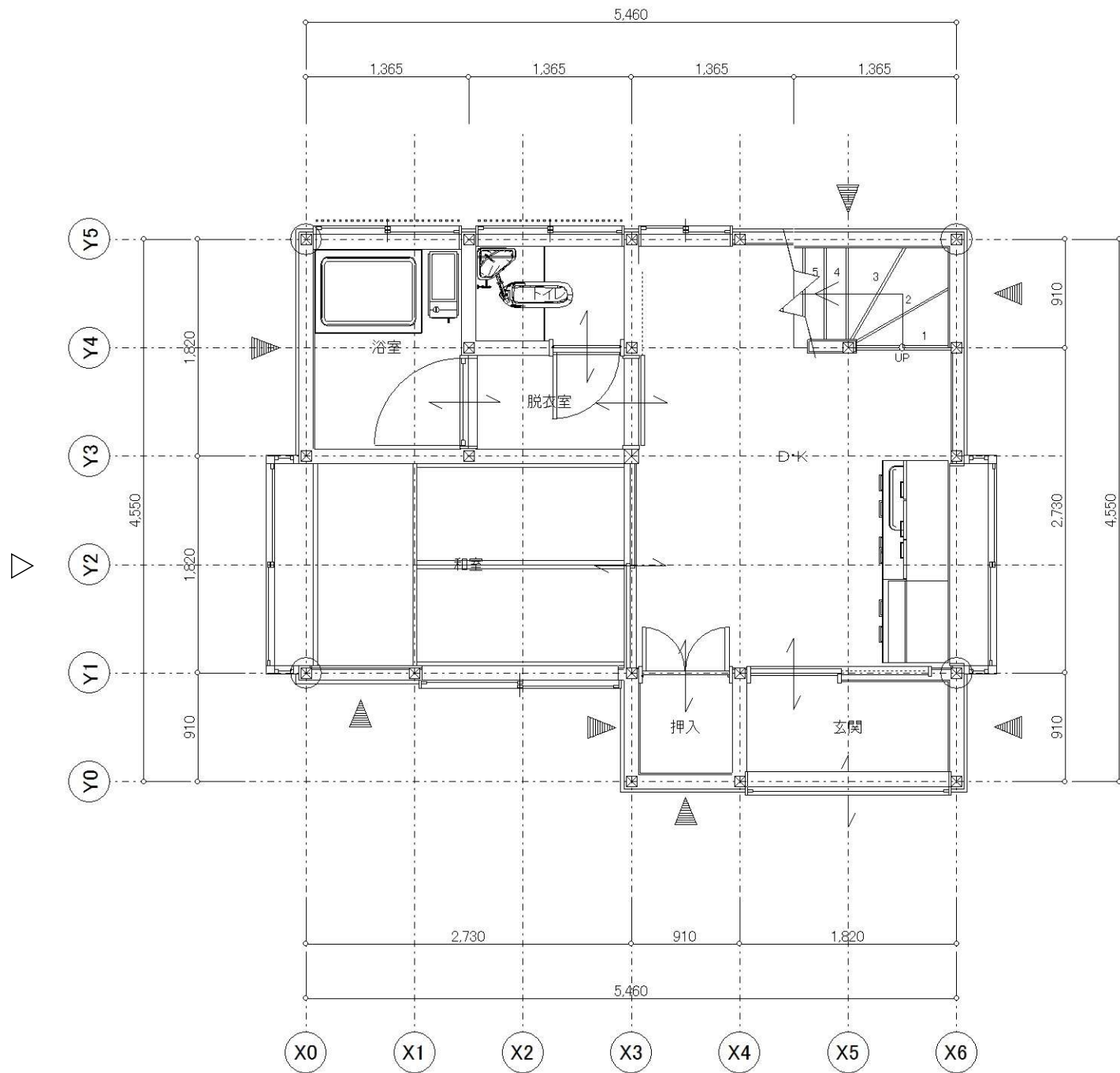
平面図-1F
