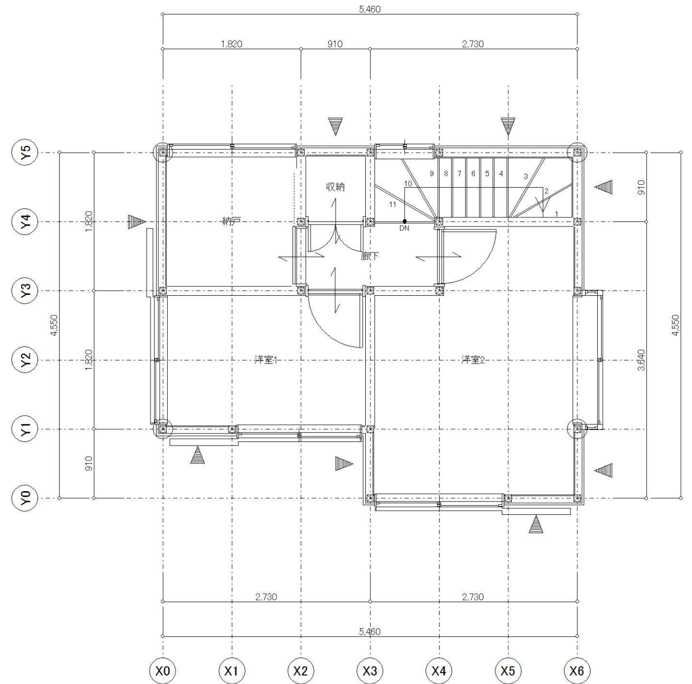
平面図-2F
