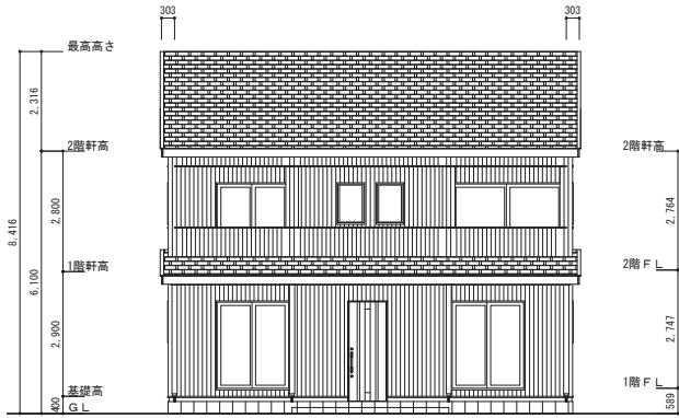
南侧 立面图 S : 1/100
