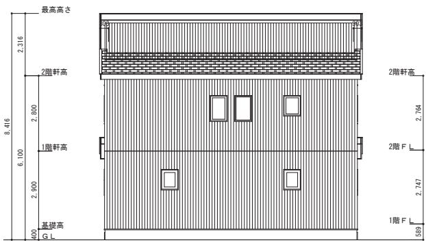
北侧 立面图 S : 1/100
