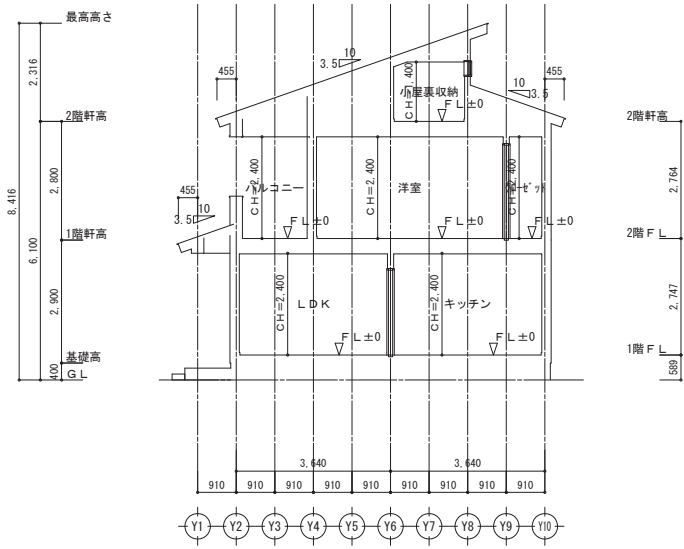
1面 断面図 S : 1/100
