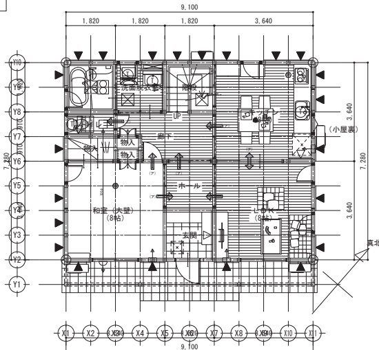
1F 平面図 S : 1/100
