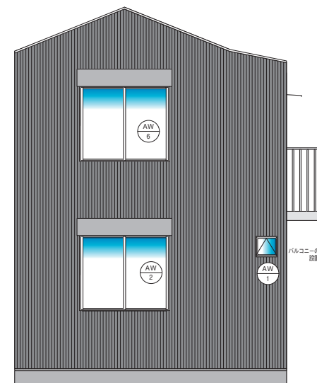
西側立面図
