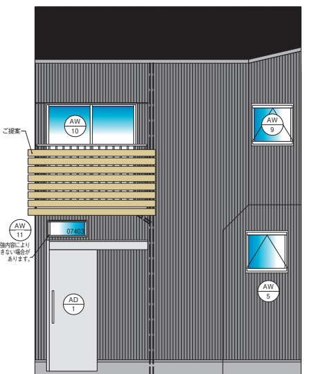
南側立面図
