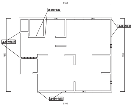
リフォーム前(耐震補強前)
