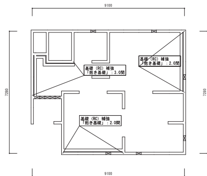
リフォーム後(耐震補強後)
