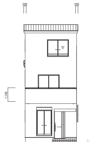
北侧立面图
