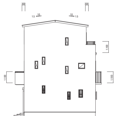
西侧立面图
